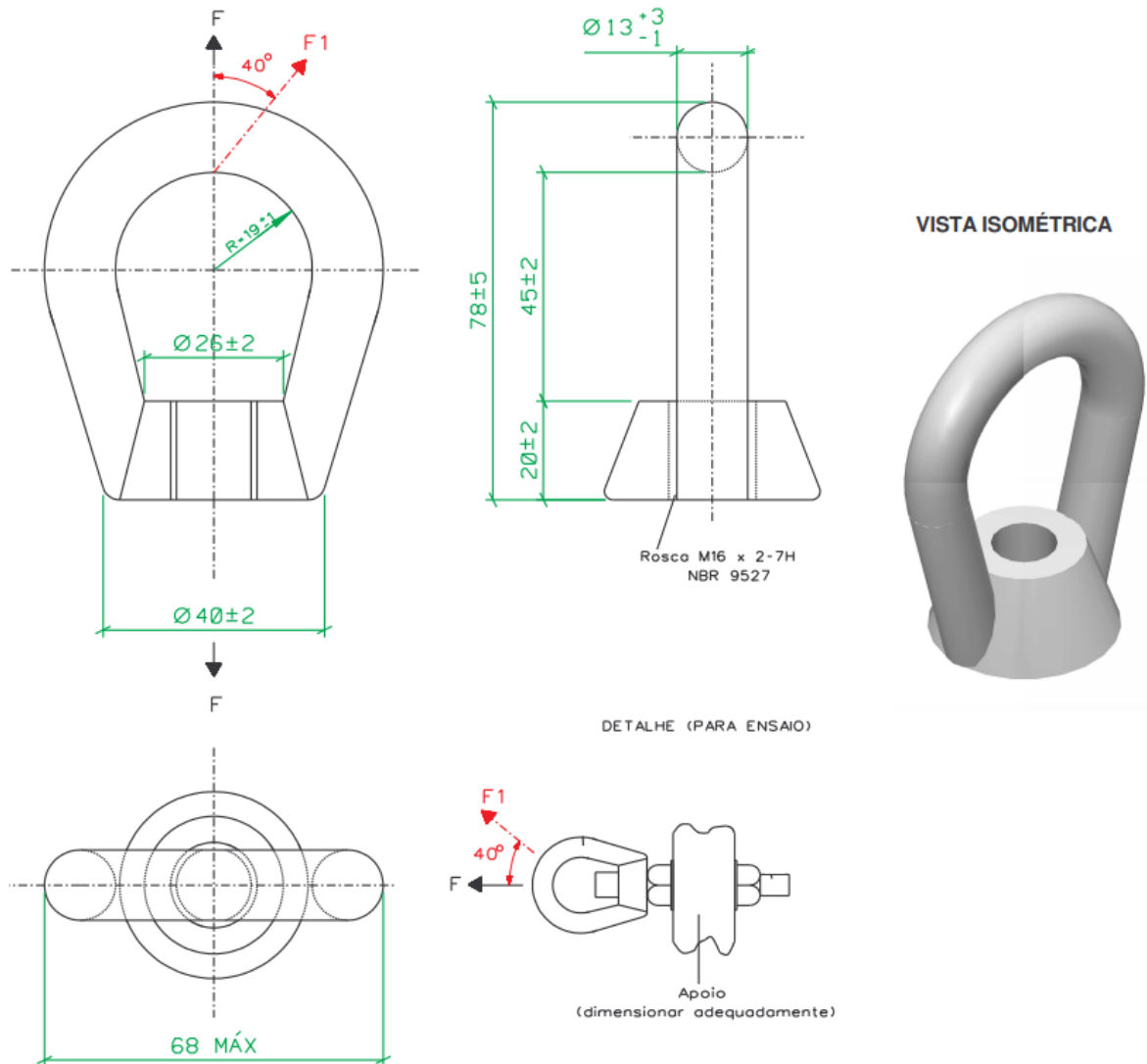
FIGURA 1 – Porca olhal
