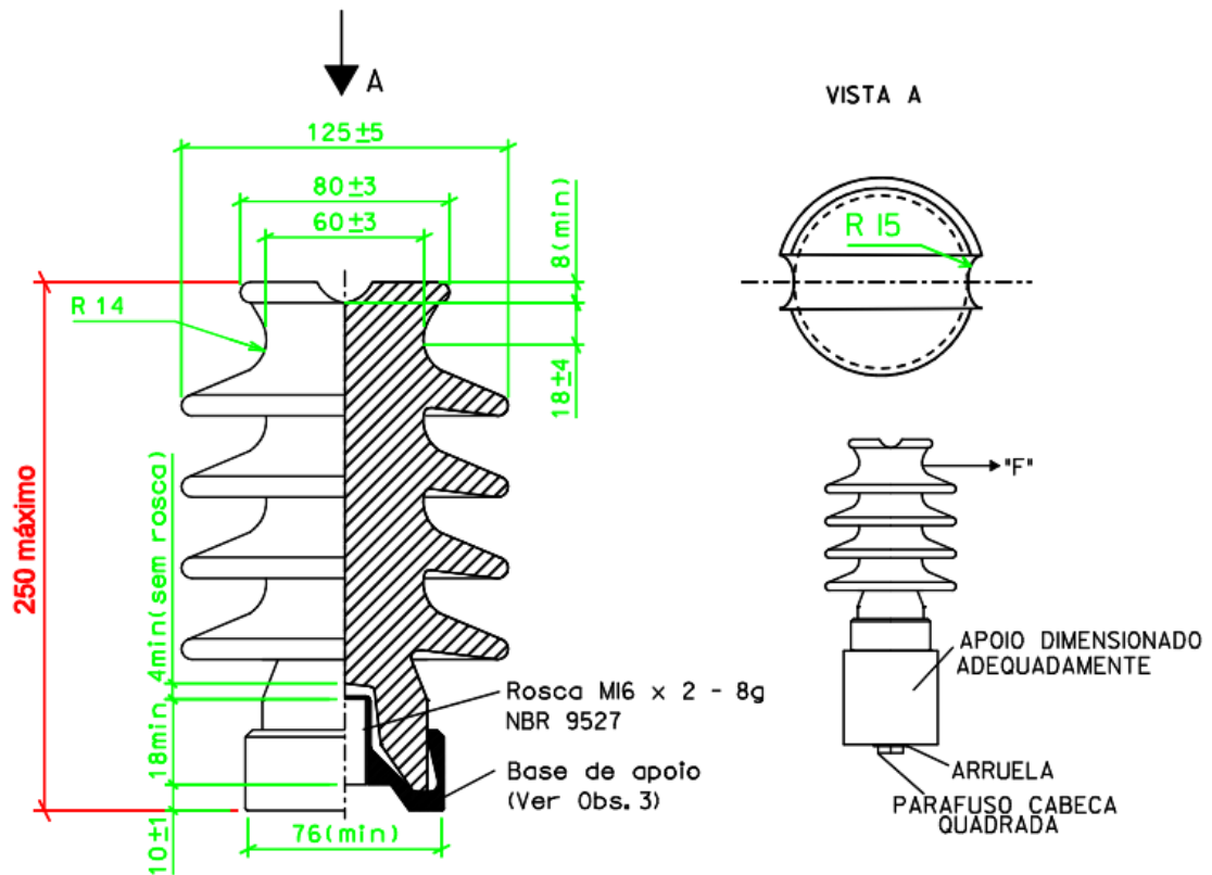
FIGURA 1 – Isolador tipo pilar 13,8kV
