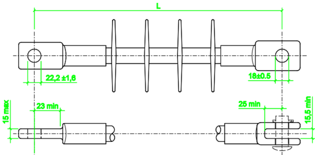
FIGURA 1 – Isolador de ancoragem tipo bastão 36,2kV
