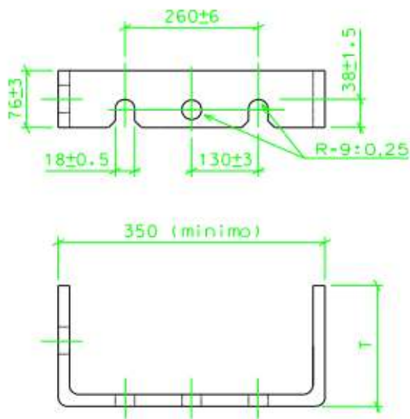
FIGURA 12 – Suporte para fixação do transformador monofásico no poste
