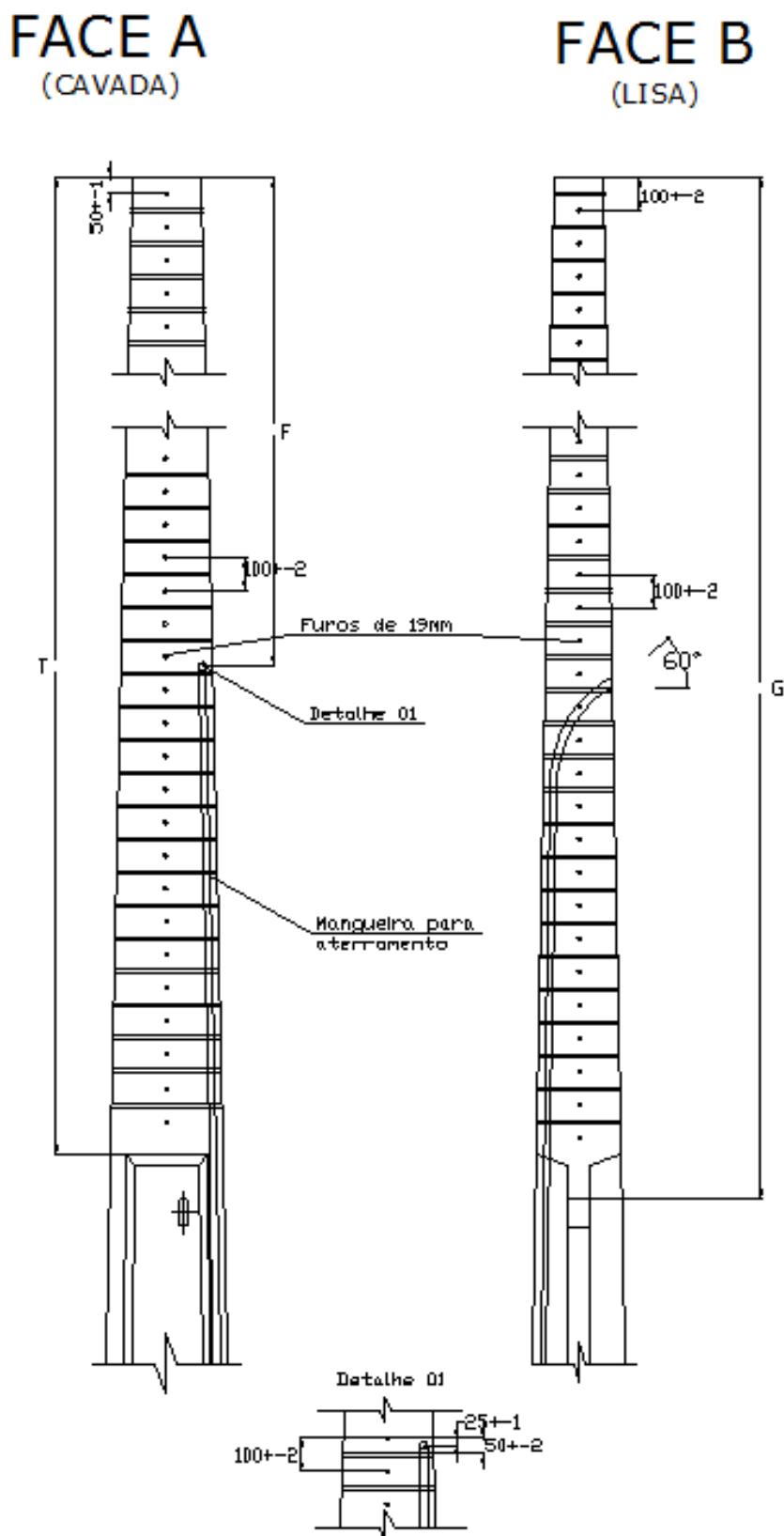
FIGURA 2 – Detalhes do topo do poste
