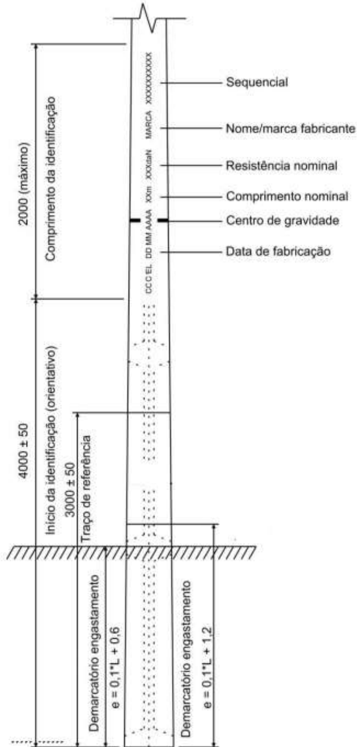
FIGURA 3 - Identificação dos postes duplo T
