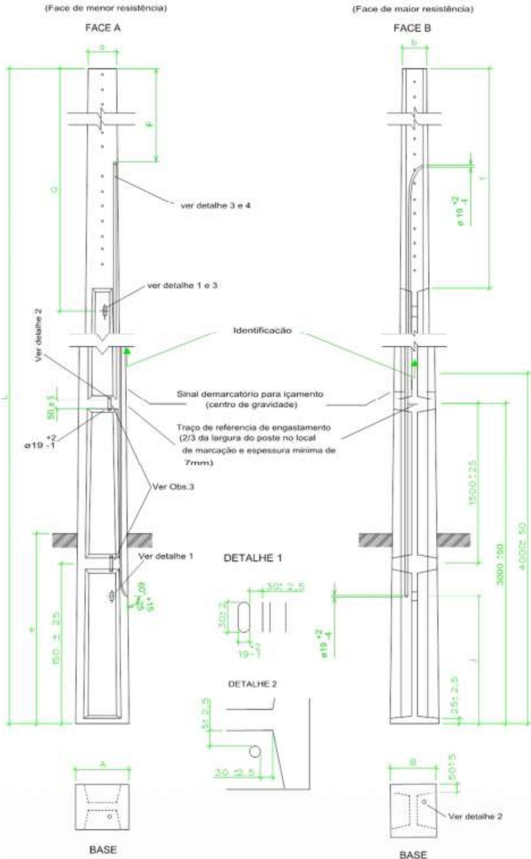
FIGURA 1 – Dimensões dos postes duplo T
