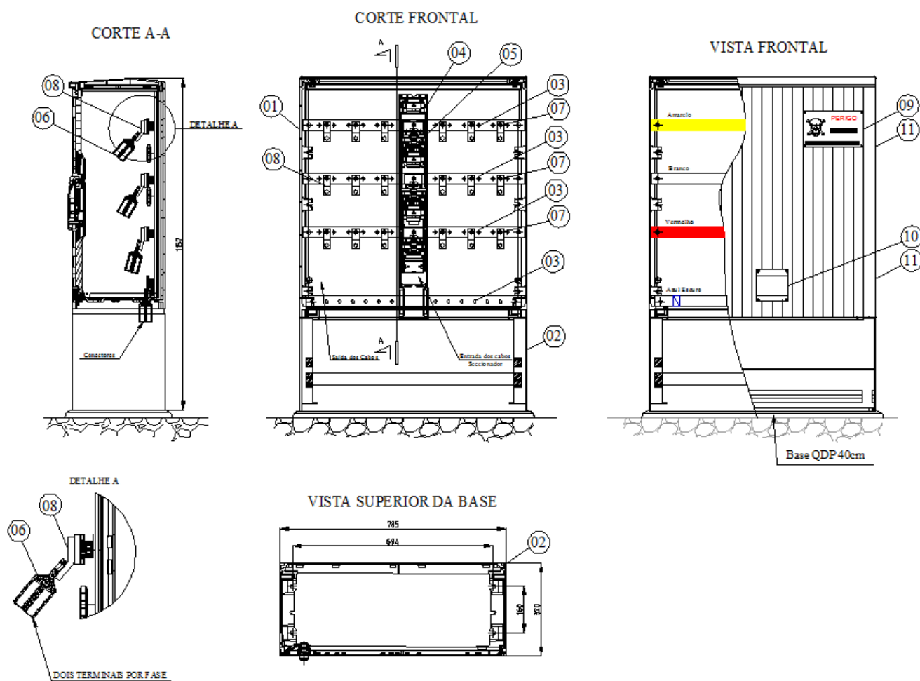
Figura 6 - Quadro de Distribuição Pedestal DIN-1 ESP
