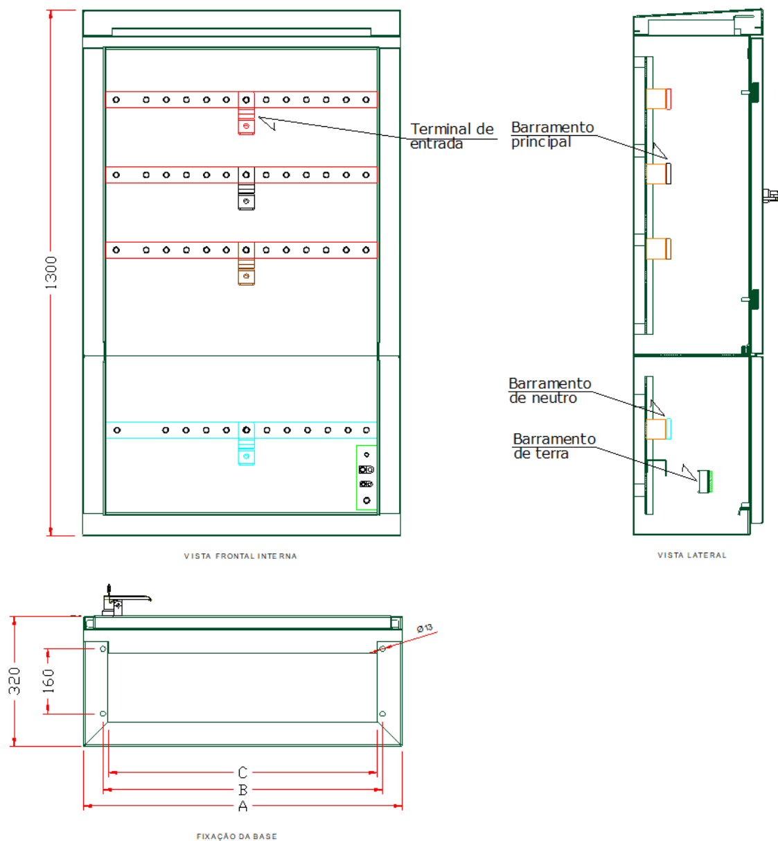
Figura 2- Quadro de Distribuição Pedestal
