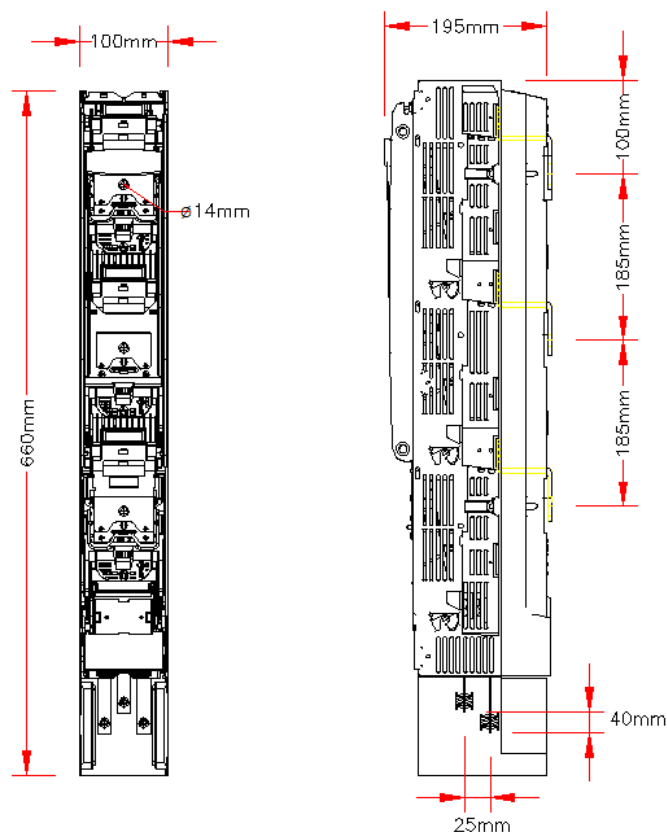
Figura 4 - Seccionadora vertical abertura tripolar
