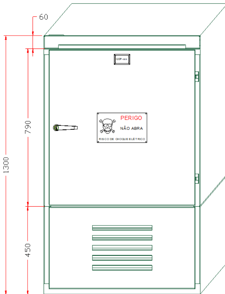
Figura 1- Quadro de Distribuição Pedestal Polimérico
