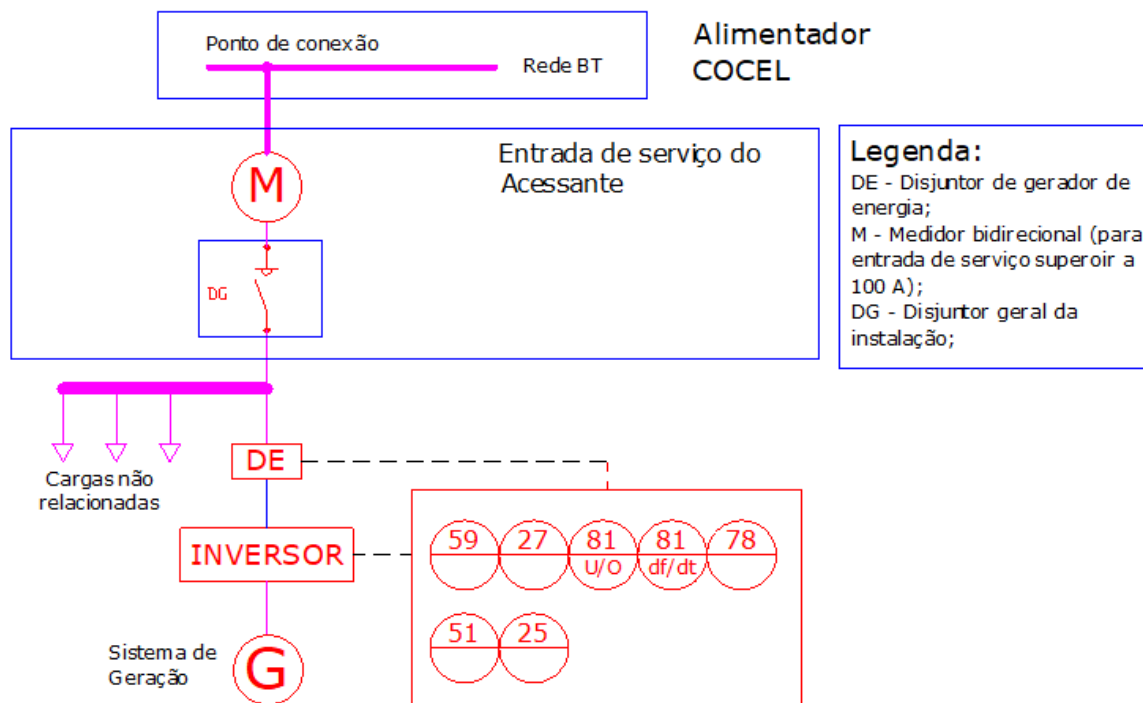
Figura 7.3 - Microgeração atendida em BT - Geração com uso de inversor.
