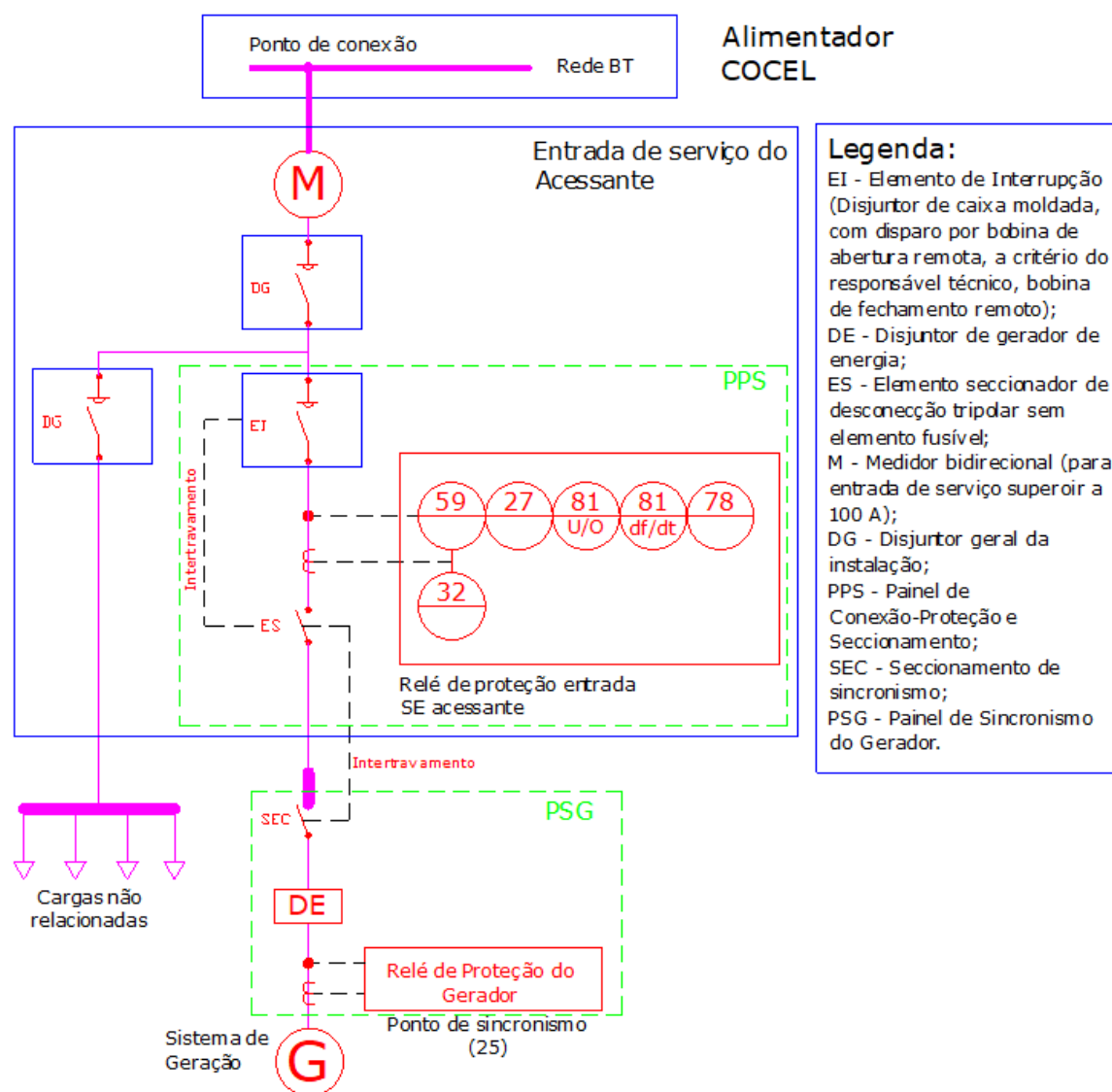
Figura 7.2 - Microgeração atendida em BT - Geração sem o uso de inversores.
