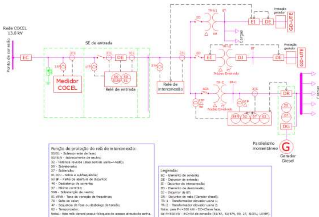
Figura 6.4 - Esquema Unifilar de UC com GD-M – Opção do EI na MT e na BT
