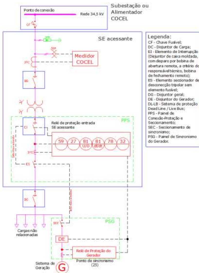
Figura 7.22 – Microgeração em 34,5 kV – Geração até 75 kW na BT com TF maior que 300 kVA.
