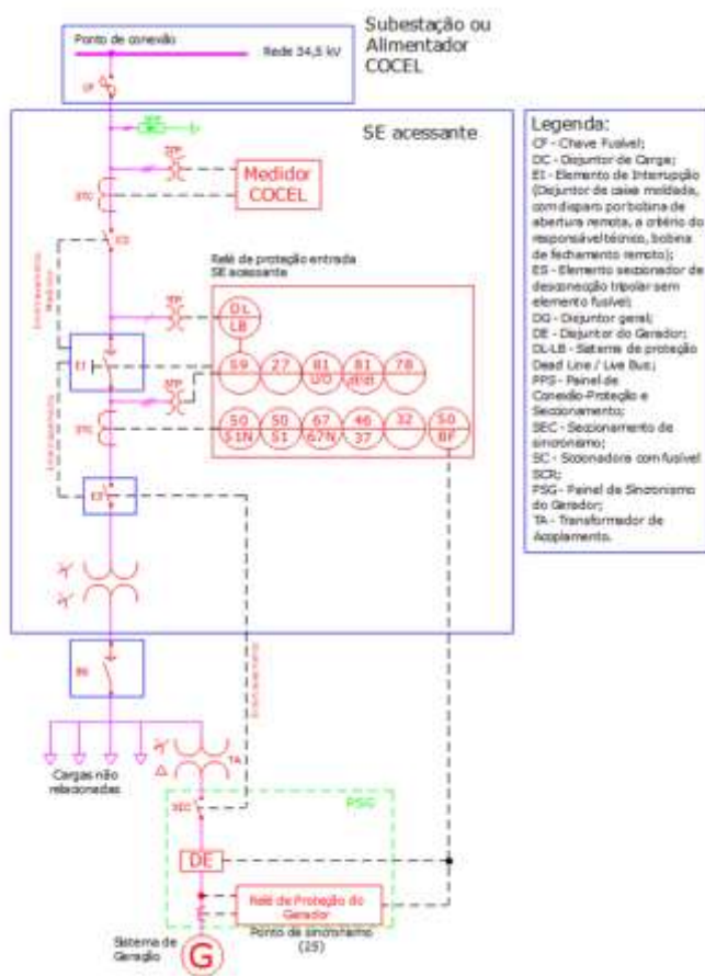
Figura 7.27 – Minigeração atendida em 34,5 kV – acima de 300 kW até 500kW - Geração sem o uso de inversores.
