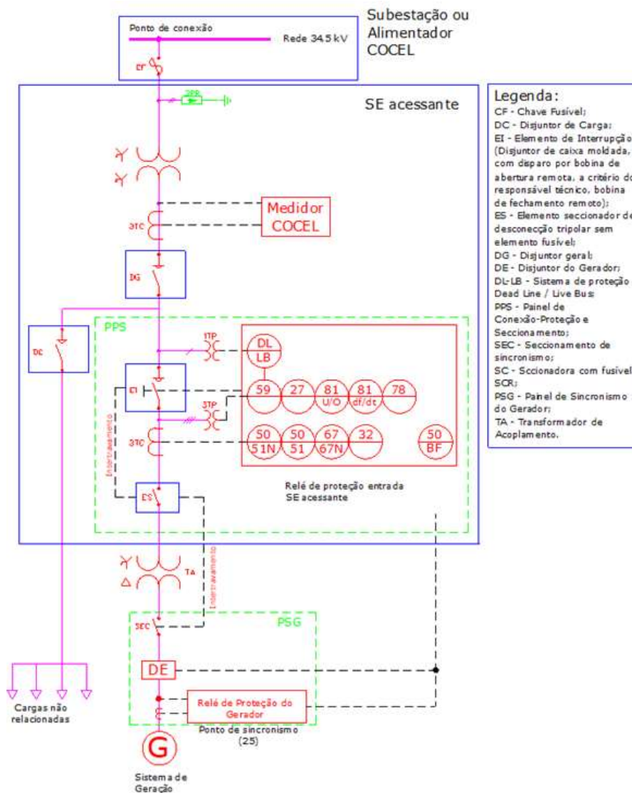
Figura 7.25 – Minigeração em 34,5 kV – acima de 75 kW até 300kW - Geração sem o uso de inversores.
