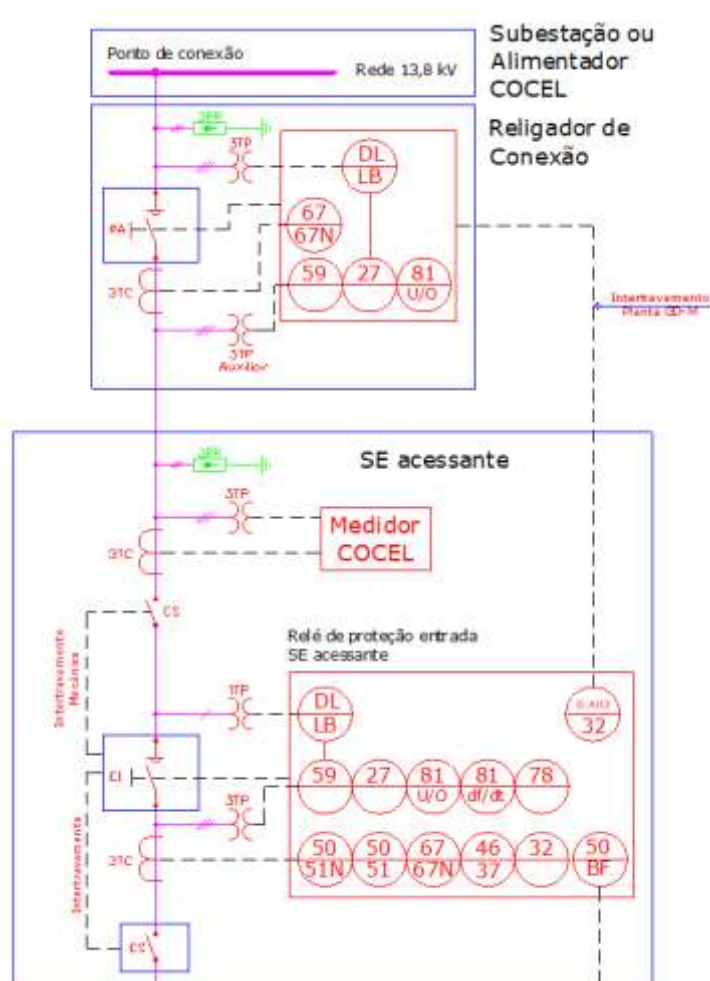
Figura 6.13 – Intertravamento entre RA de Conexão com Relé do Disjuntor EI
