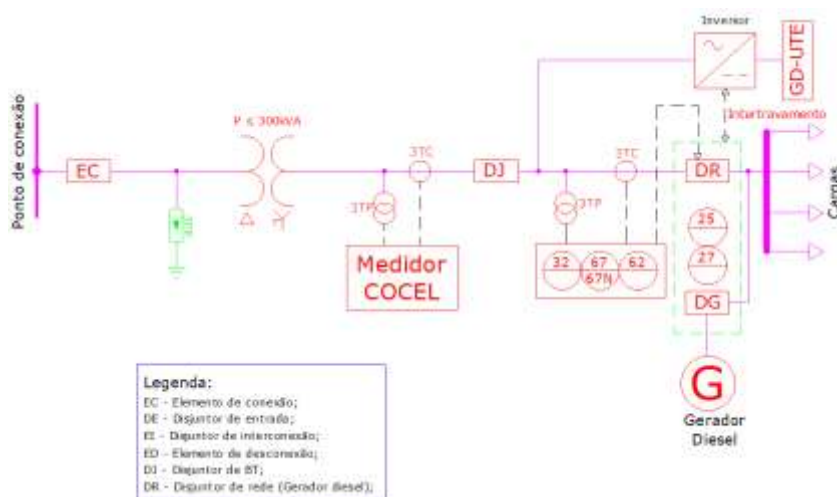
Figura 6.14 – Diagrama Unifilar Simplificado de Conexão GD e Geração com PM na BT
