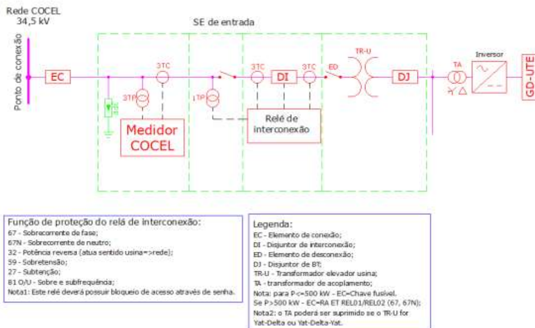
Figura 6.10 – Conexão de UFV em planta GD-S
