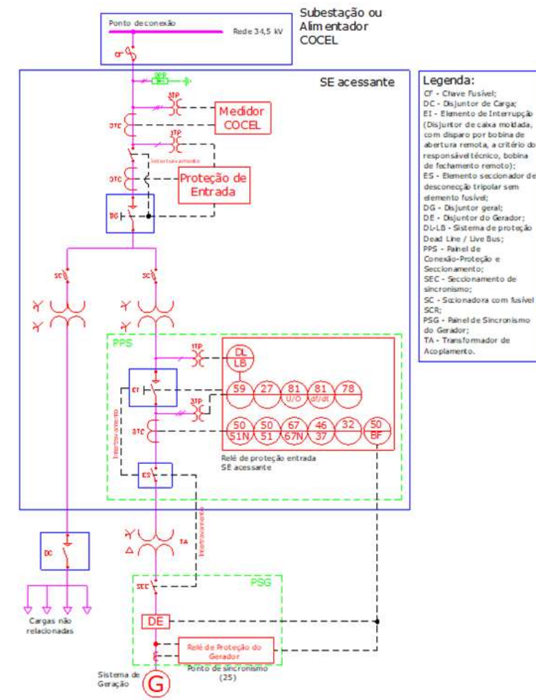
Figura 7.30 – Minigeração atendida em 34,5 kV – acima de 300 kW até 500kW - Transformador Exclusivo - Geração sem o uso de inversores.
