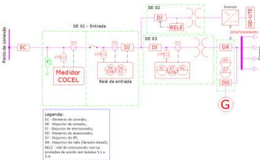
Figura 6.15 – Diagrama Unifilar Simplificado de Conexão GD e Geração com PM na MT
