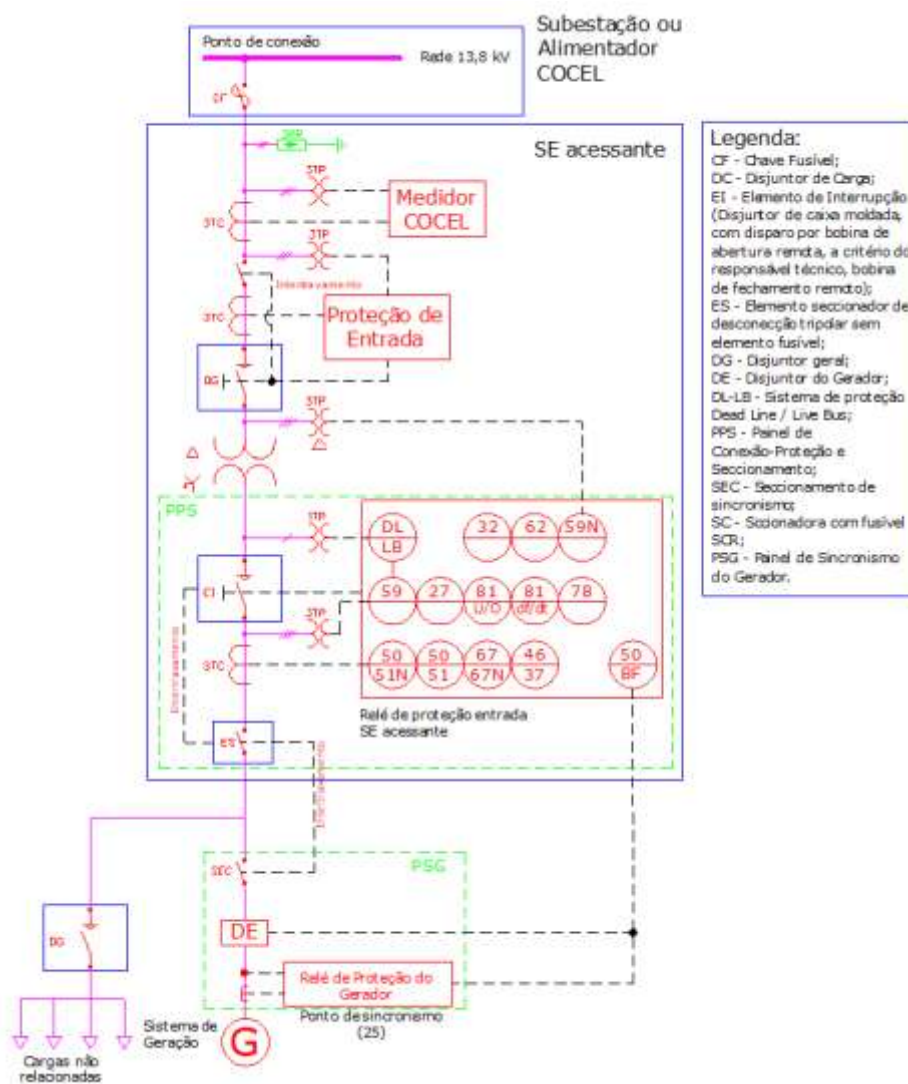
Figura 7.12 - Minigeração em 13,8 kV – acima de 300 kW até 500 kW – Geração sem o uso de inversores.
