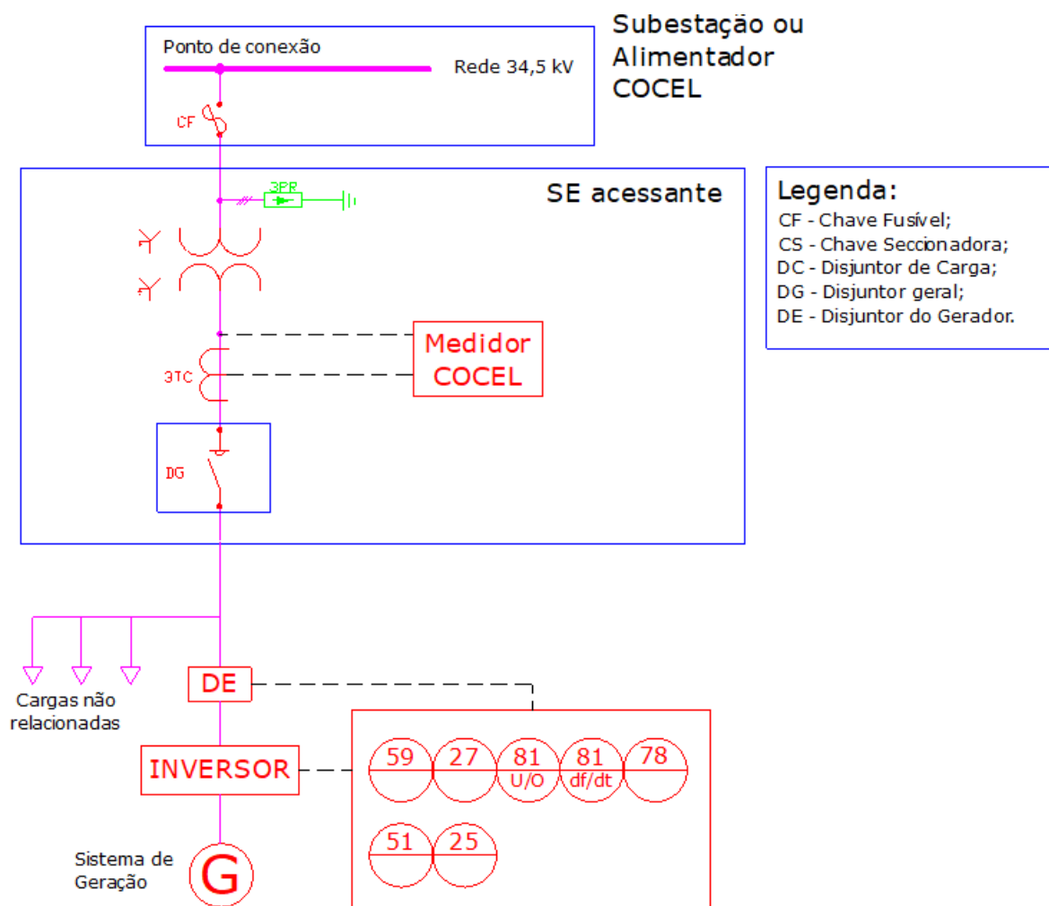
Figura 7.26 – Minigeração em 34,5 kV – acima de 75 kW até 300kW - Geração com o uso de inversores.
