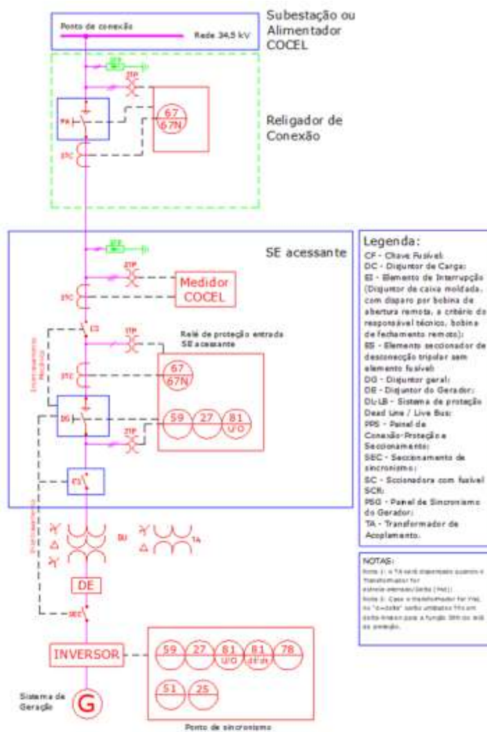
Figura 7.36 – Mini geração com o uso de inversores.
