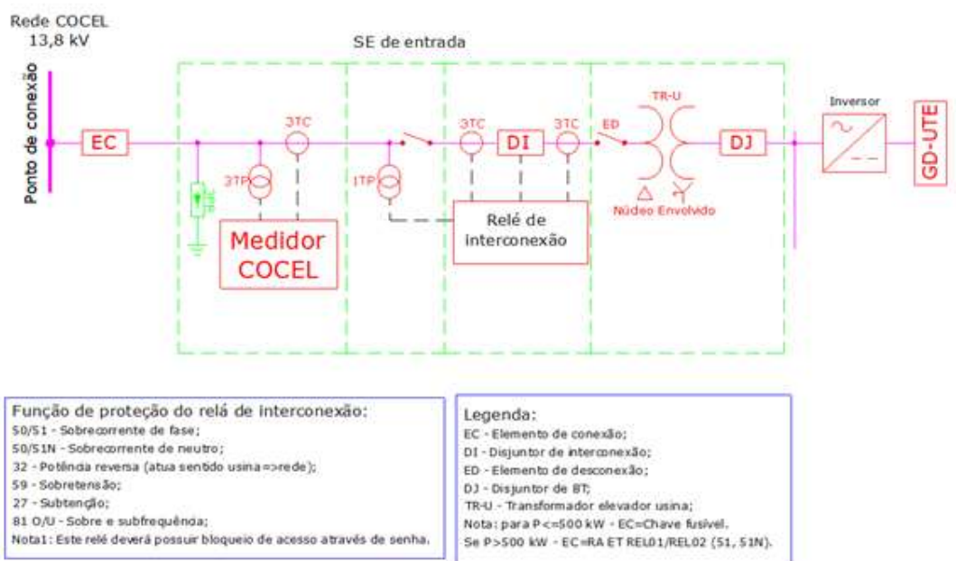
Figura 6.8 – Conexão de FV em planta GD-S
