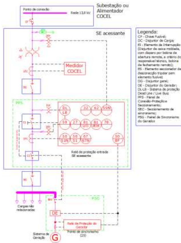
Figura 7.7 - Minigeração atendida em 13,8 kV – acima de 75 kW até 300 kW – Geração sem o uso de inversores.
