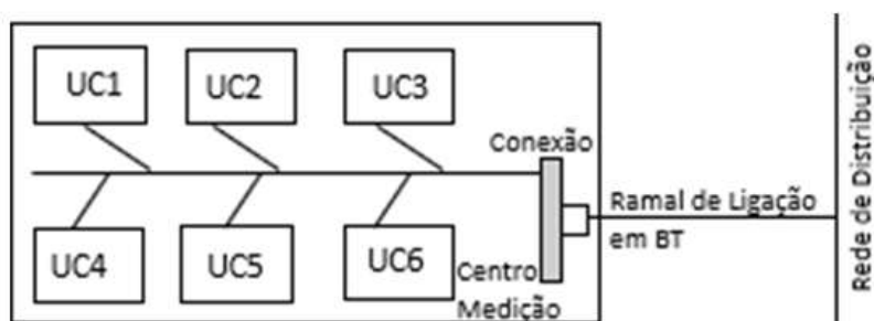
Figura 6.7 – Conexão de Micro GD que compartilham terreno
