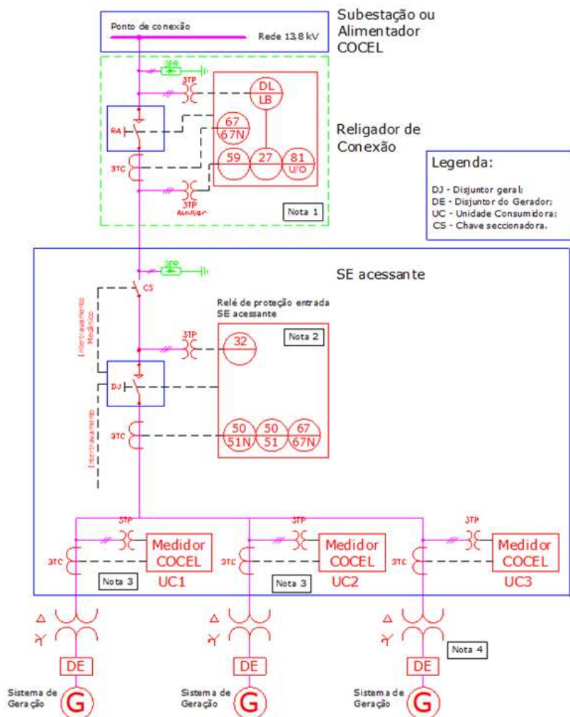
Figura 7.20 - Minigeração atendida em 13,8 kV – acima de 300 kW até 5000 kW (ou 3000 kW UFV).
