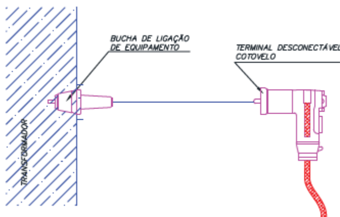
FIGURA 6 – Ligação de transformadores em pedestal com acessórios desconectáveis
