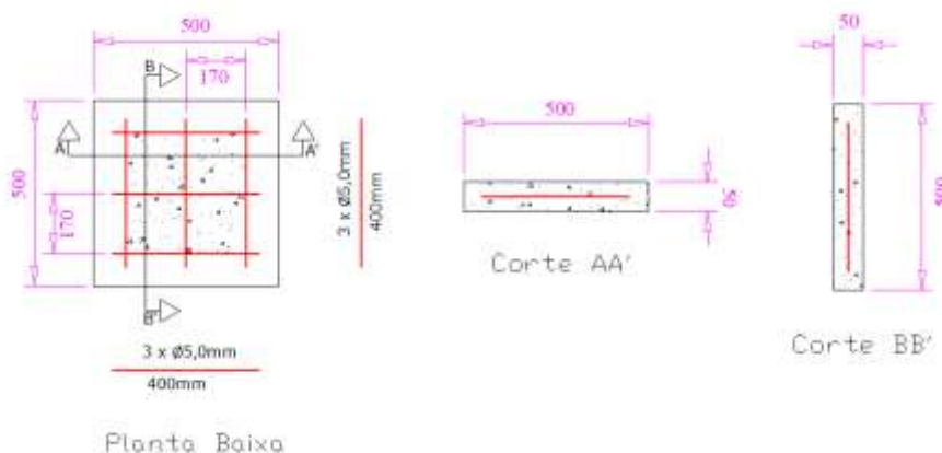
FIGURA 9 – Placa de proteção
