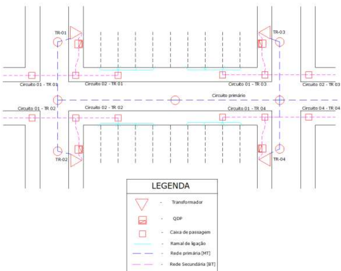
FIGURA 3 - Circuito secundário radial sem recurso
