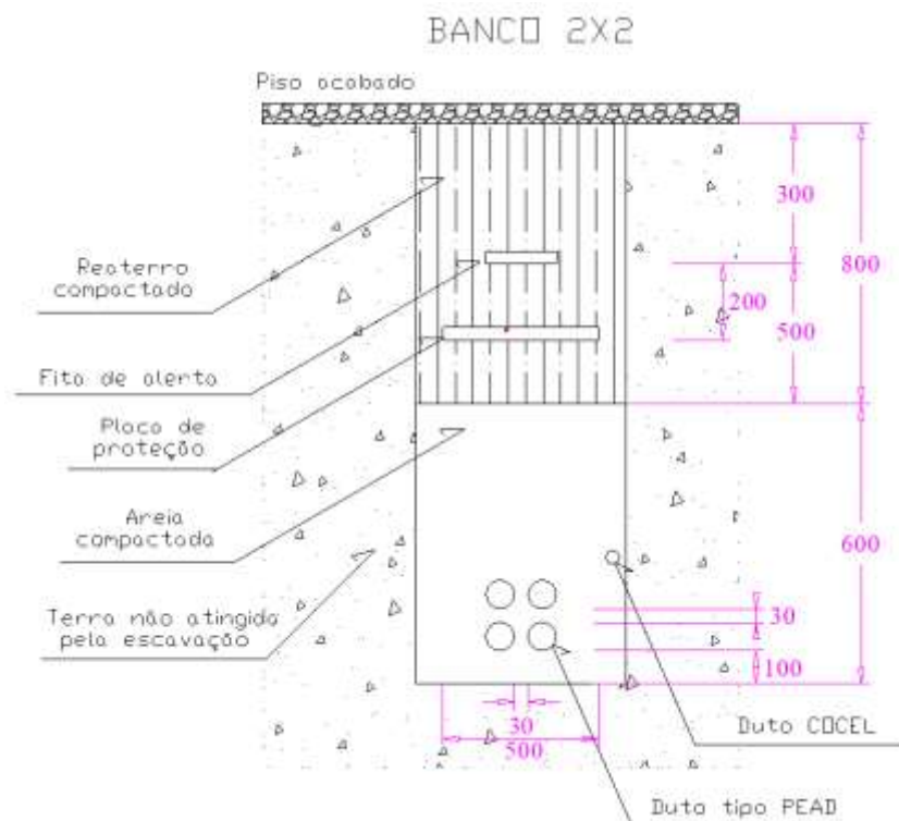
FIGURA 8 – Banco de dutos diretamente enterrados rede primária
