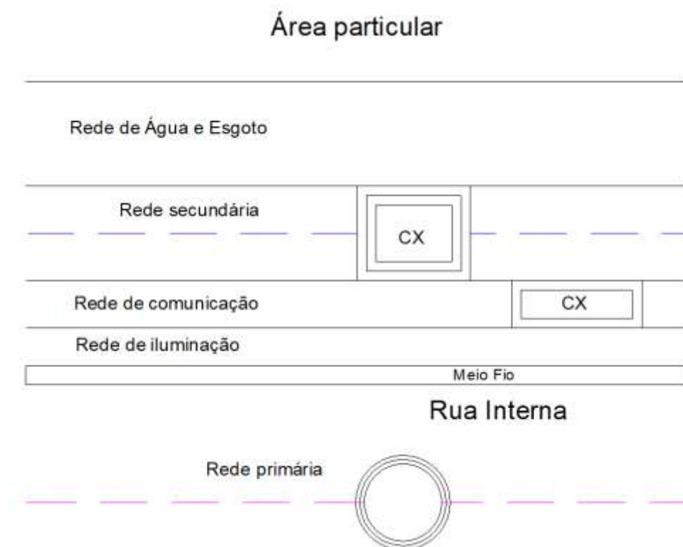
FIGURA 5 – Distribuição do banco de dutos
