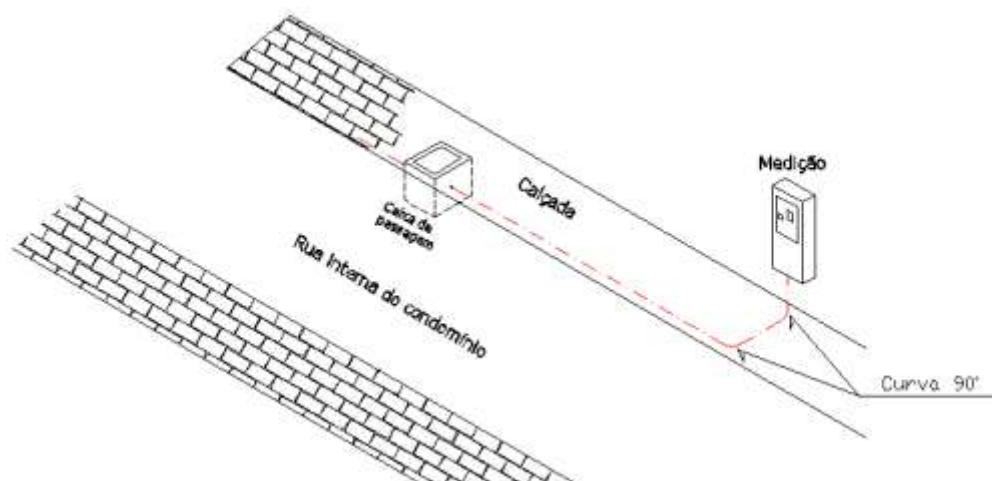
FIGURA 10 – Dutos para ramal de ligação
