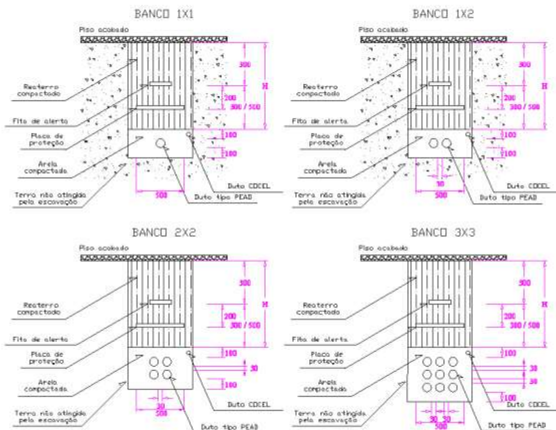
FIGURA 7 – Banco de dutos diretamente enterrados rede secundária
