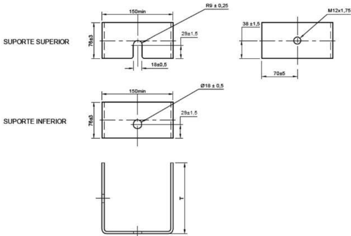
FIGURA 12 – Suporte para fixação do transformador monofásico no poste
