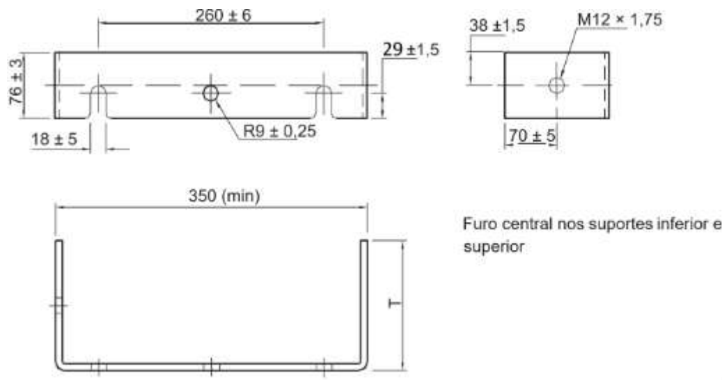
FIGURA 12 – Suporte para fixação do transformador monofásico no poste
